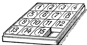
Рис. 13. Игра в 15.
